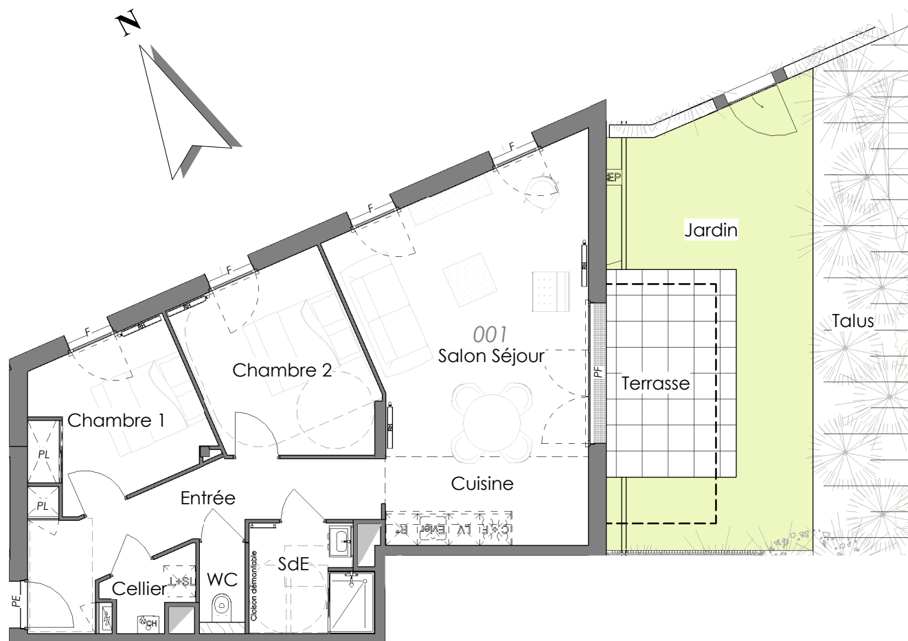
Plan du Logement 001 ( 1 : 100 )
