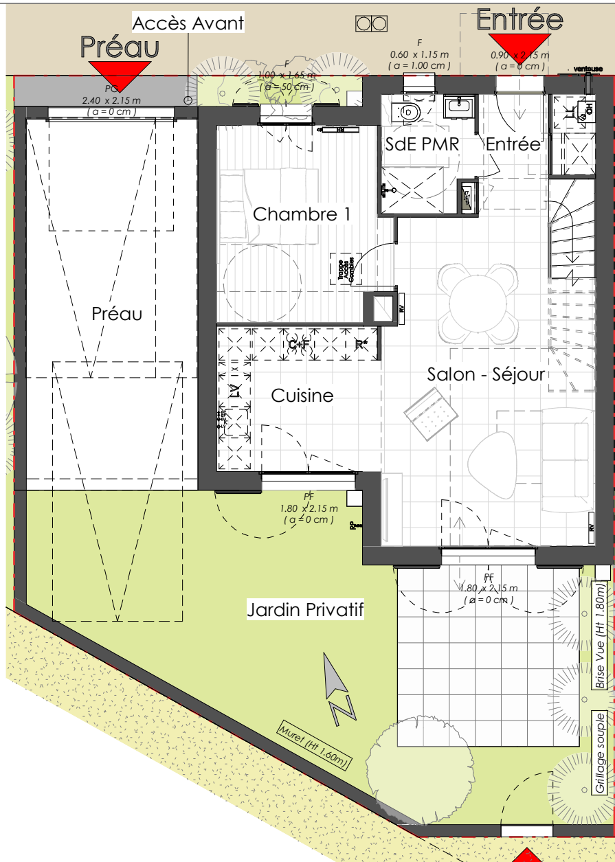
RDC (1 : 100)
