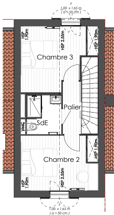
Plan de l'Etage (1 : 100)
