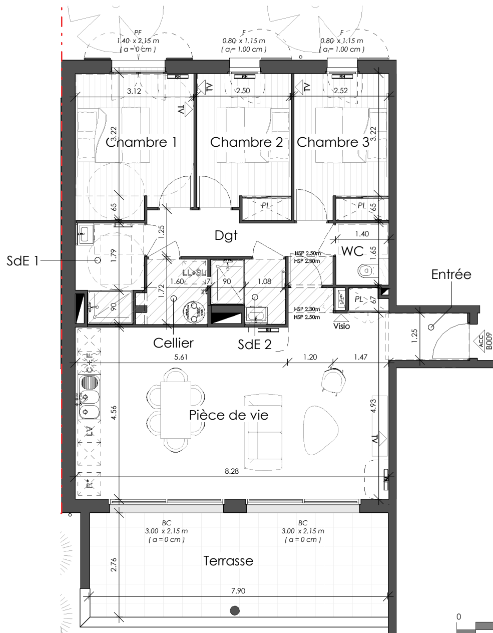
Plan du Logement ( 1 : 100 )
