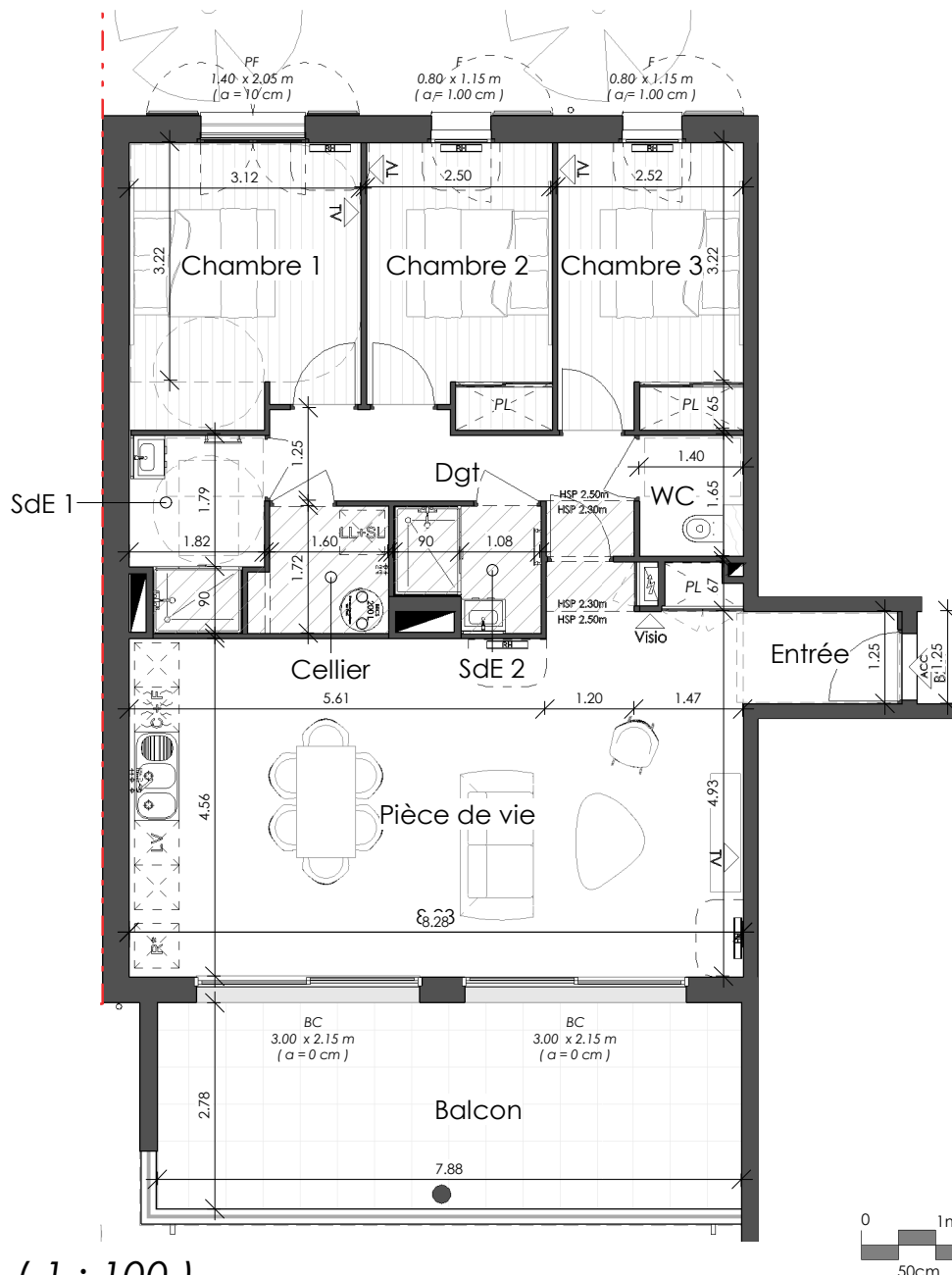
Plan du Logement (1 : 100)
