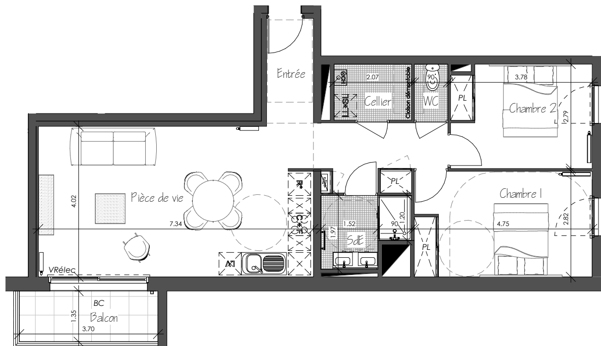
Plan de niveau du R+2 ( 1 : 100 )
