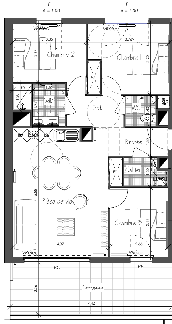
Plan de Niveau du R+3 (1 : 100)
