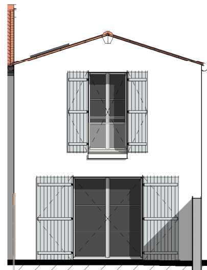
Façade Arrière ( 1 : 100 )
