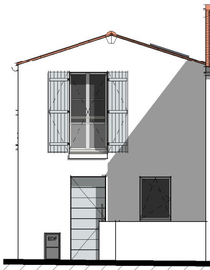
Façade Avant ( 1 : 100 )
