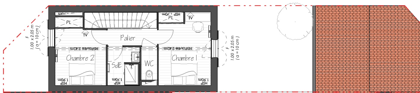
R+1 (1 : 125)
