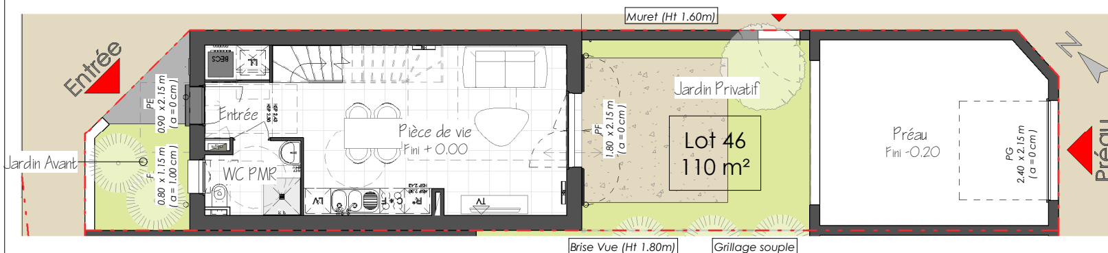
RDC (1 : 125)
