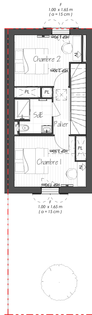
R+1 (1 : 125)
