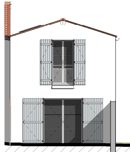
Façade Arrière ( 1 : 100 )
