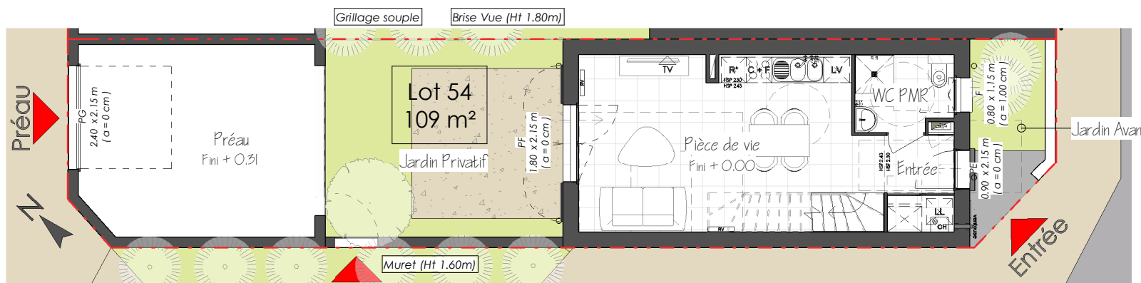
RDC (1 : 125)
