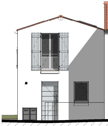
Façade Avant ( 1 : 100 )
