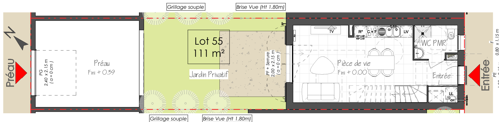
RDC (1 : 125)
