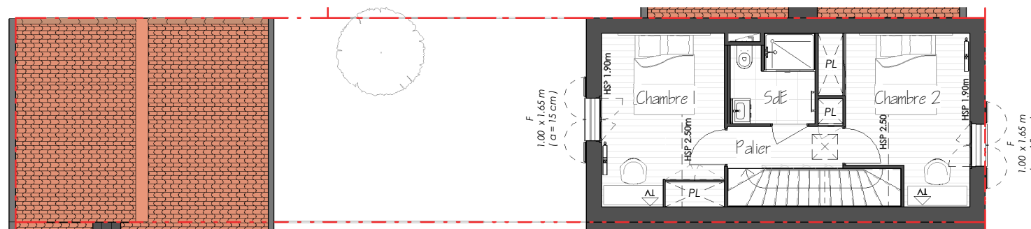
R+1 (1 : 125)
