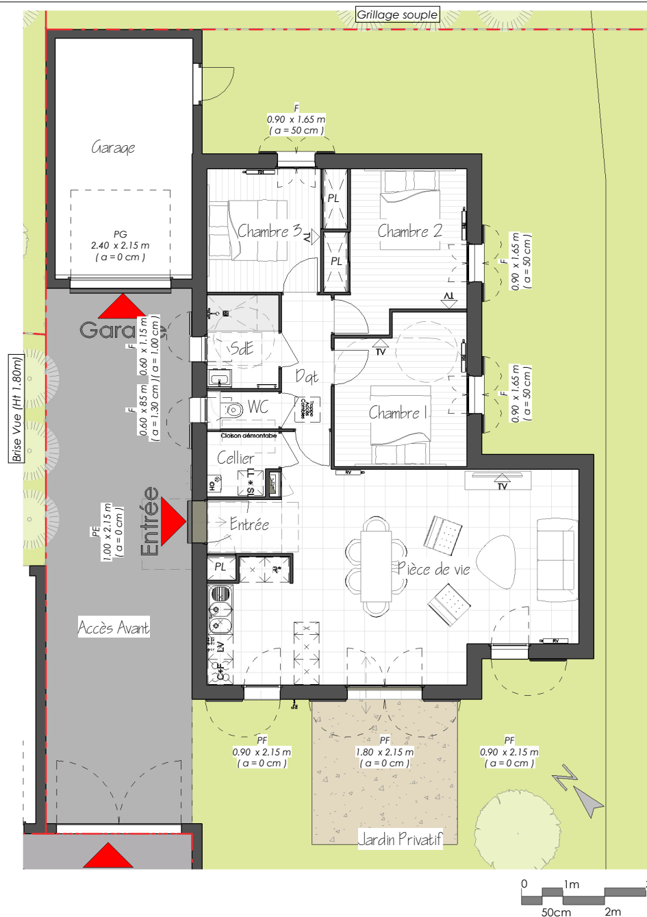
RDC (1 : 125)
