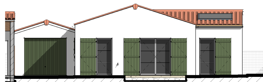
Élévation Sud-Ouest (1 : 125)
