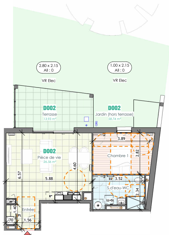
Plan du logement D002 (1 : 150)
