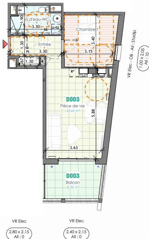
Plan du logement D003 (1 : 150)
