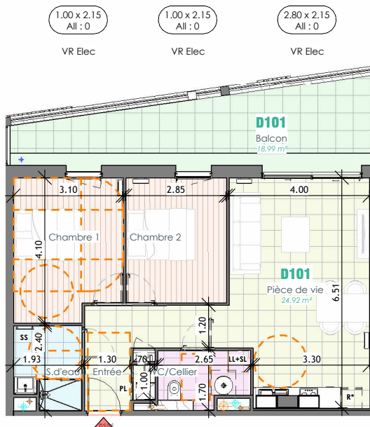
Plan du logement D101 (1 : 150)
