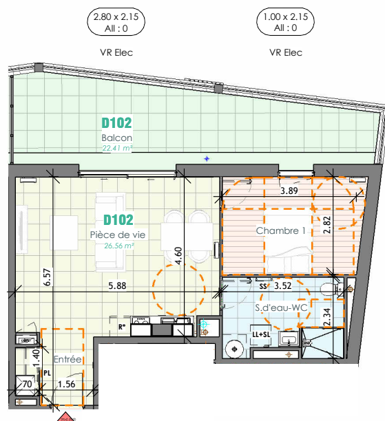
Plan du logement D102 (1 : 150)
