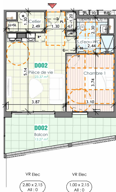
Plan du logement D002 (1 : 150)
