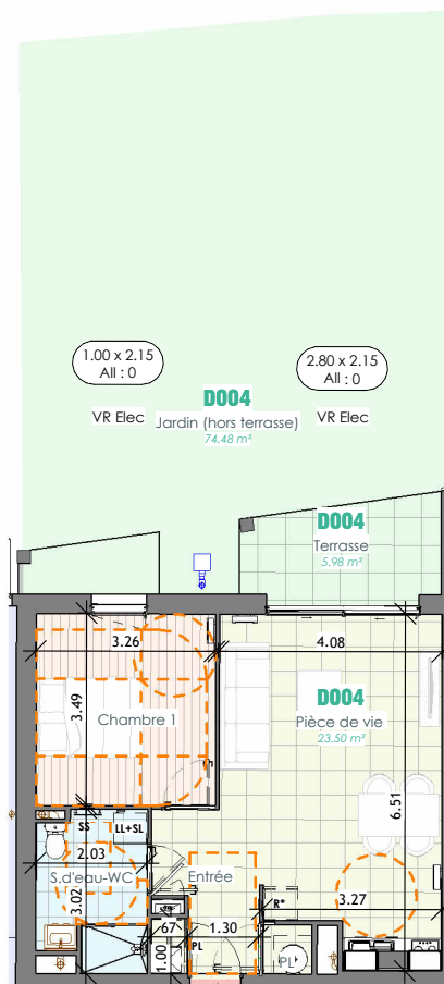
Plan du logement D004 (1 : 150)
