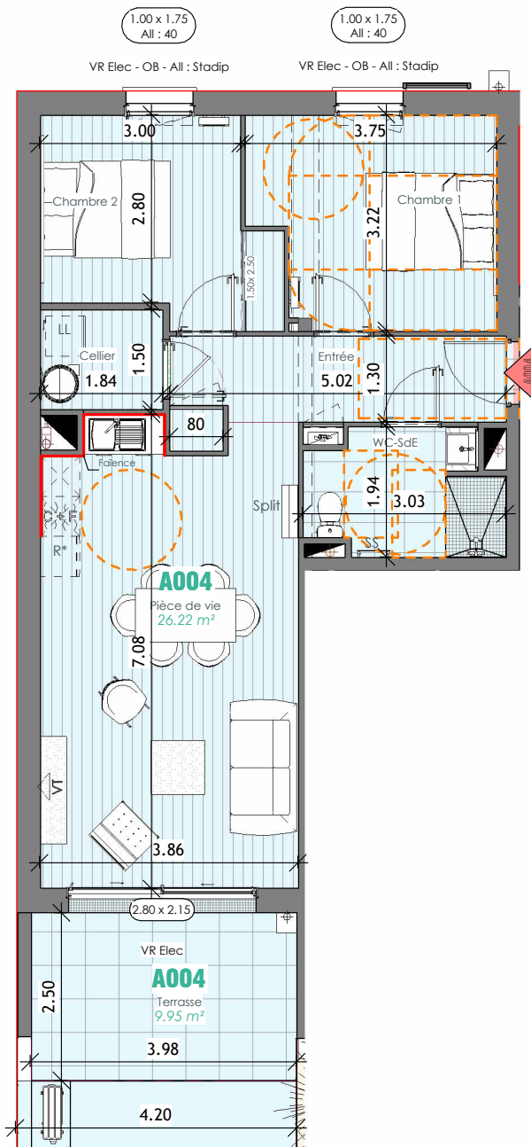
Plan du logement A004 Ech : 1 : 100
