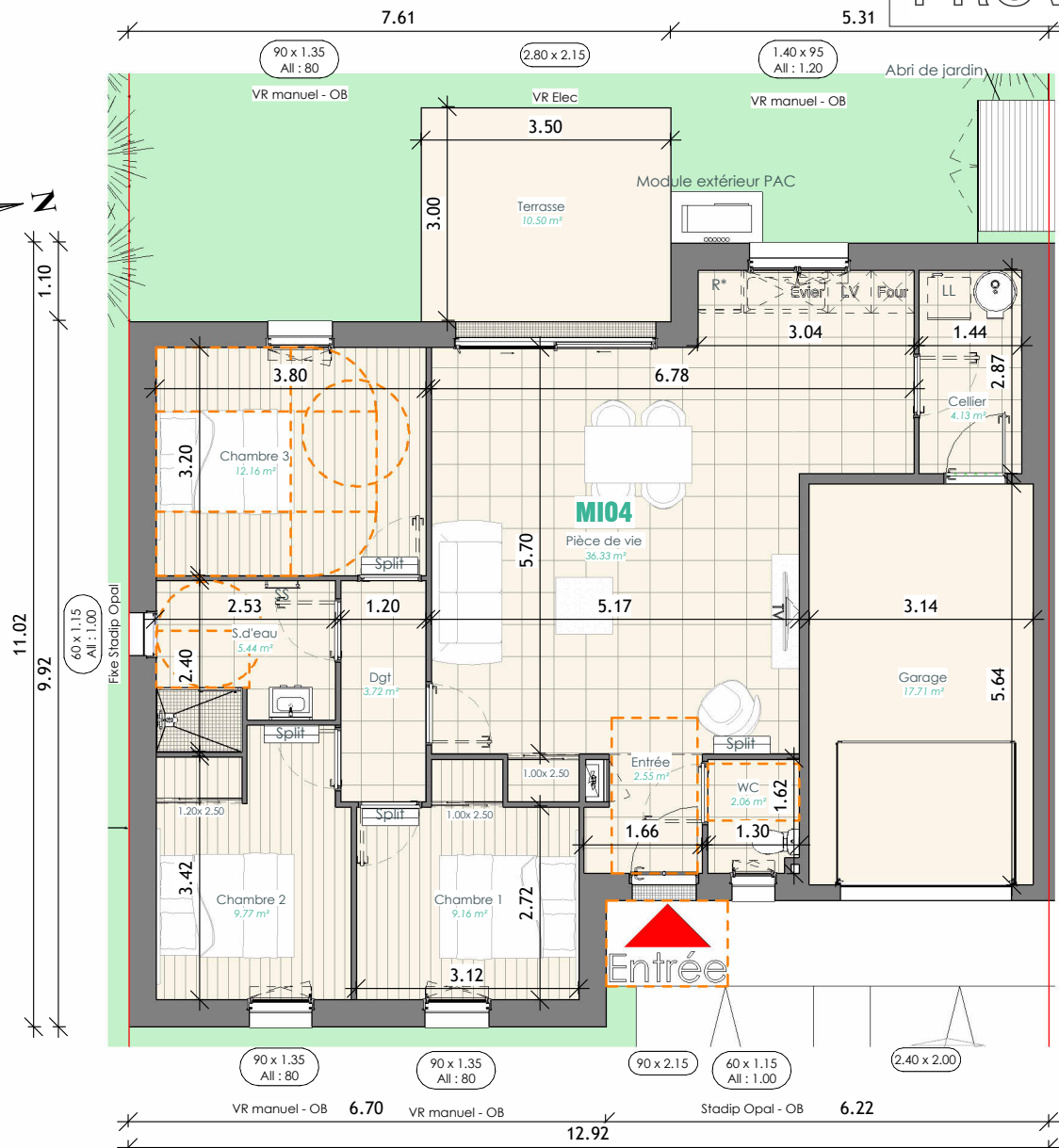
RDC MI04 Ech : 1 : 100
